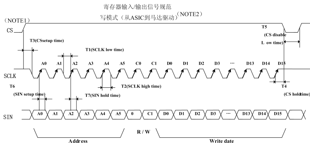
图 1. 写数据模式
