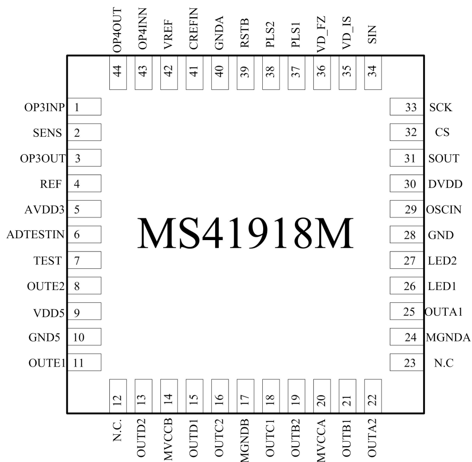
管脚排列图
